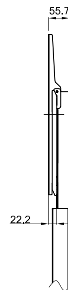
TV取り付け金具位置(S=1:10)
